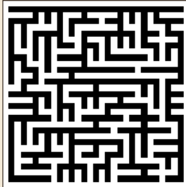
Sidewinder
