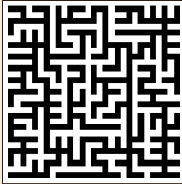
Sidewinder
