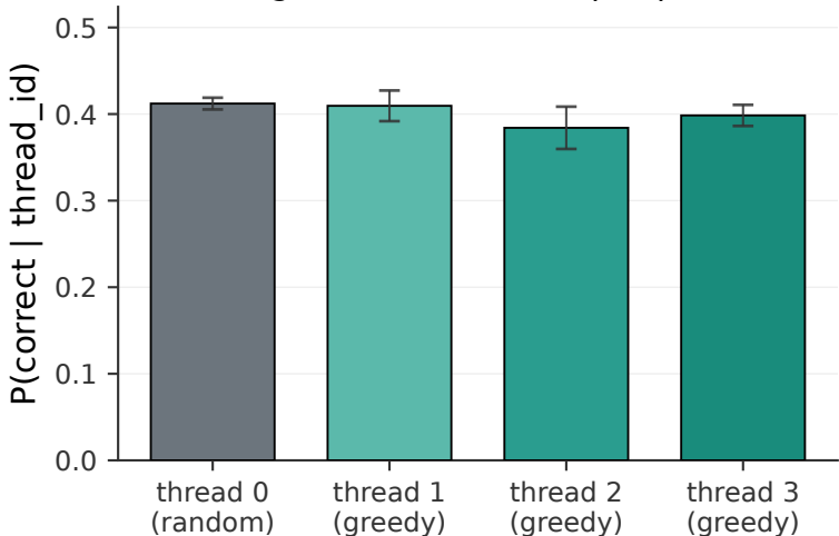
gemma3-12b x hotpotqa
