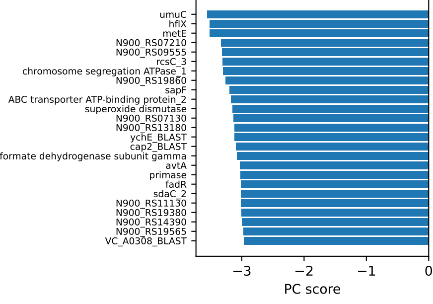
PC6 negative genes
