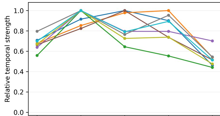
PCA
