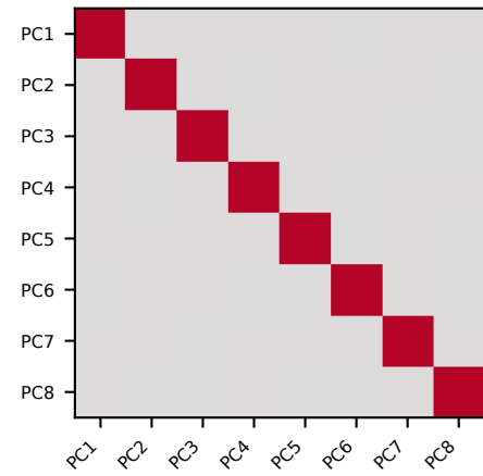
PCA
