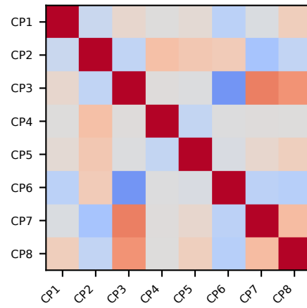
CP
