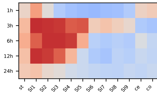
PCA 1
