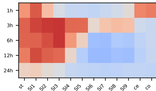
PCA 2
