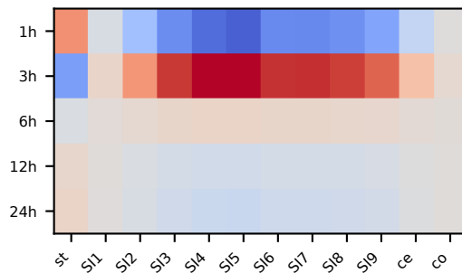
CP 2
