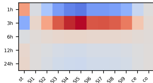
CP 2
