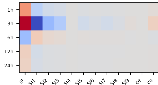
CP 3
