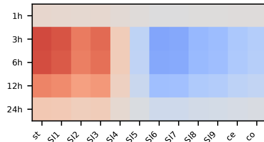
CP 1
