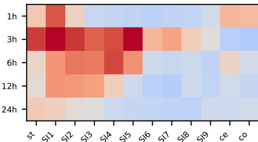
PCA 3
