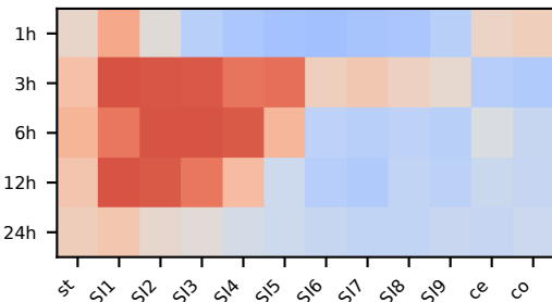
PCA 1
