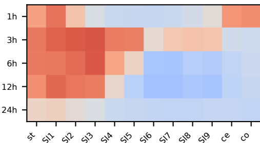
PCA 2
