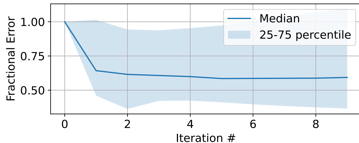
Parameter d
