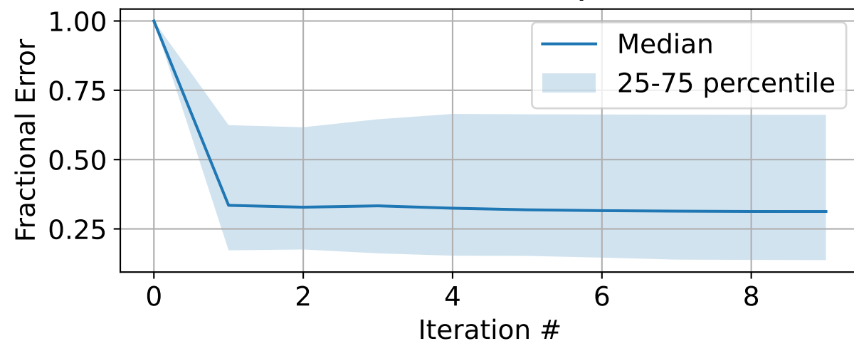
Parameter Q
