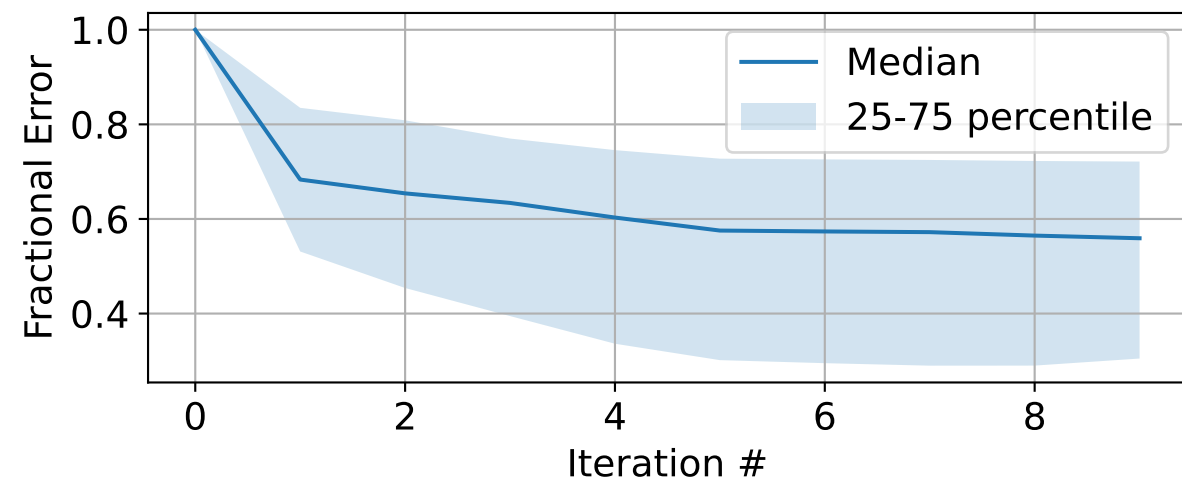
Parameter d
