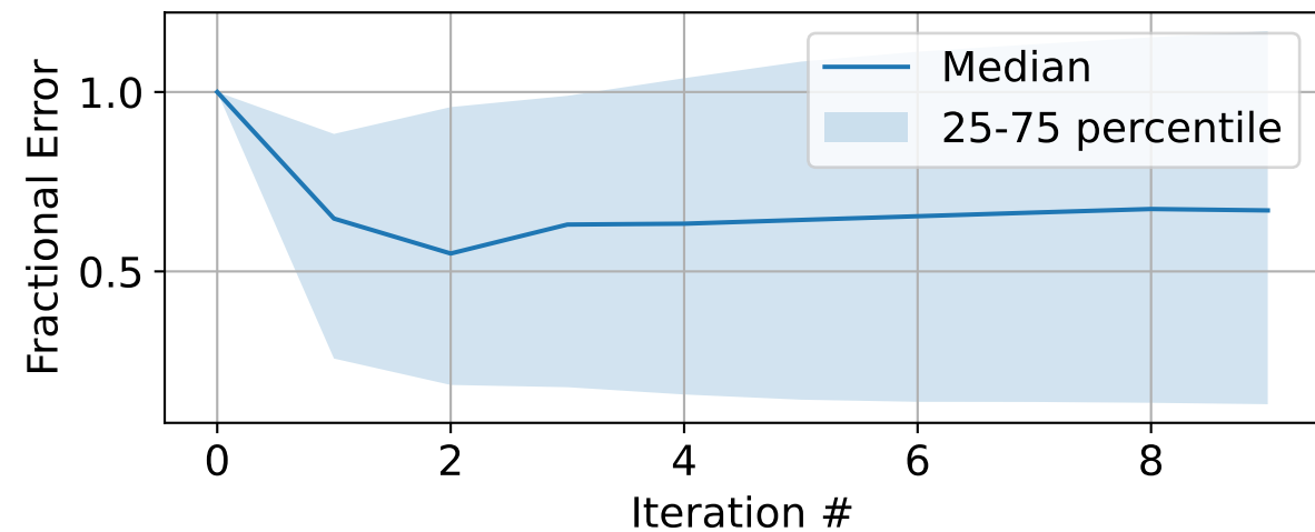
Parameter b
