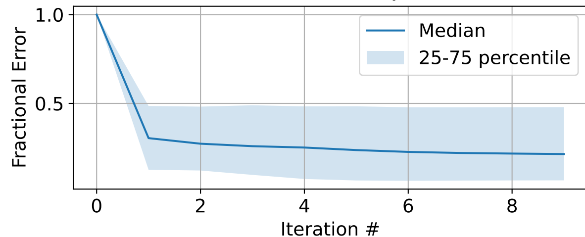
Parameter Q
