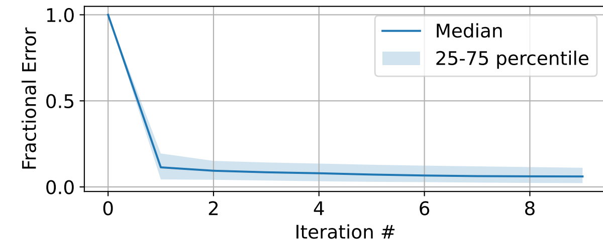
Parameter P
