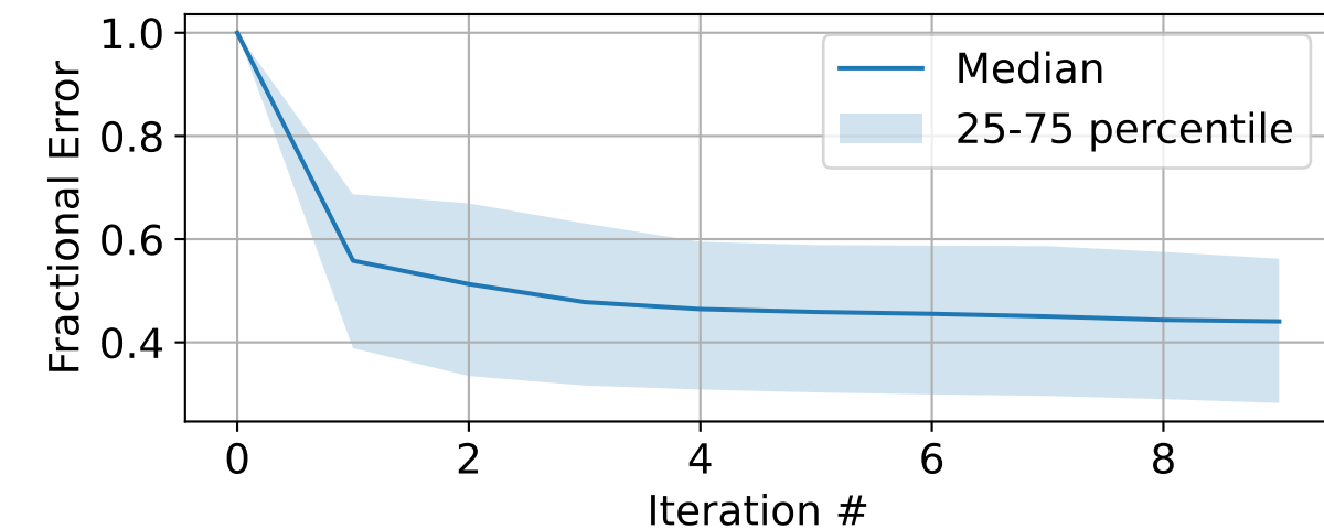
Parameter c
