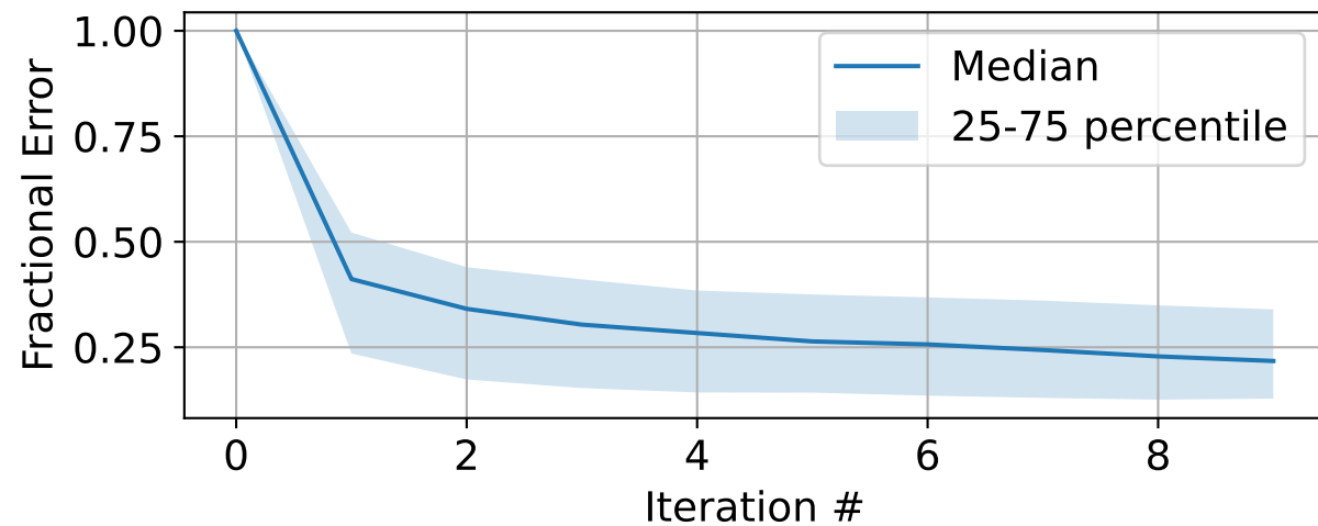
Parameter a
