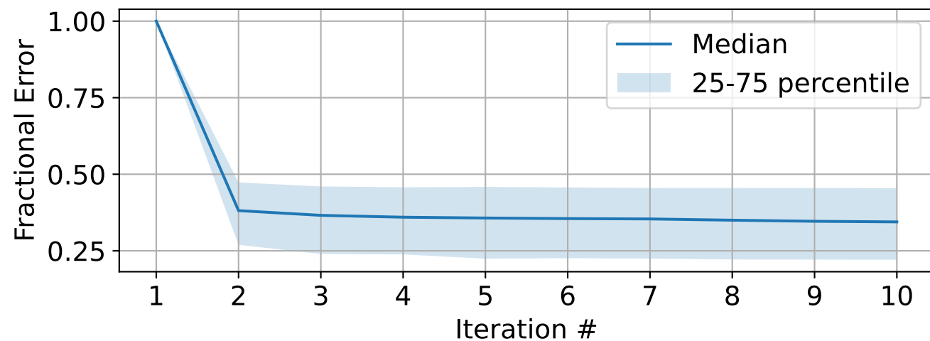
Parameter c
