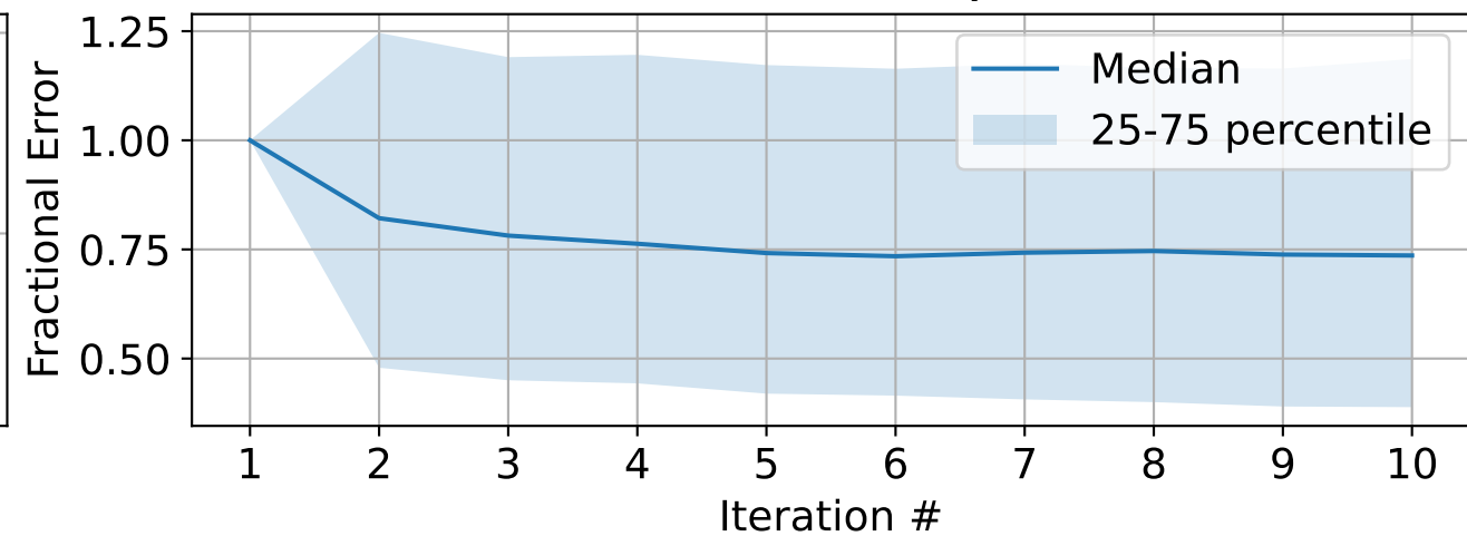
Parameter Q
