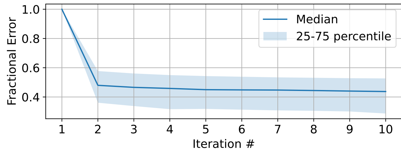
Parameter d
