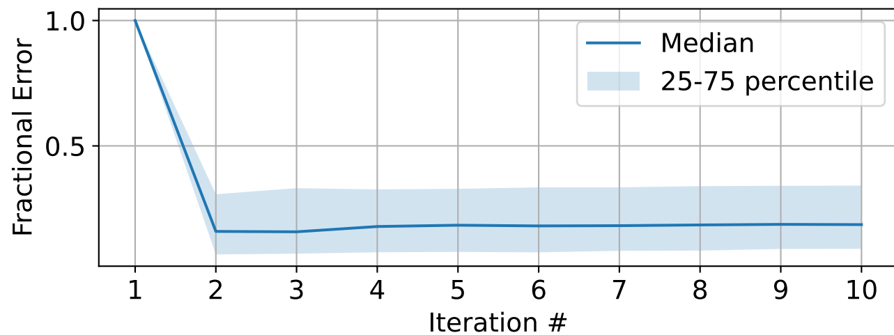
Parameter P
