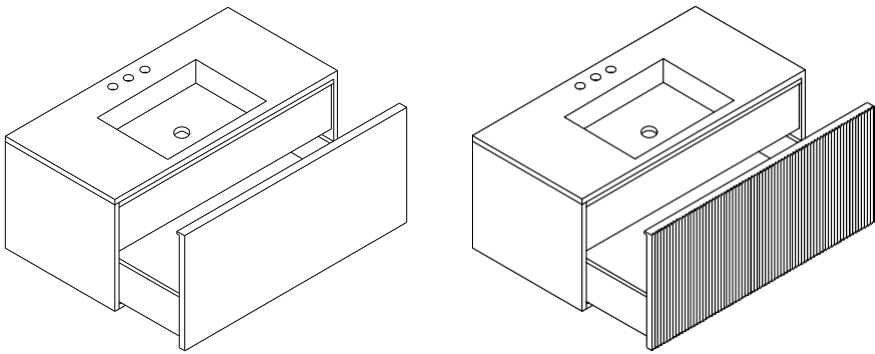
MODULARE SOSPESO CON LAVABO INTEGRATO L90H40 DECK-MOUNTED TAPWARE (3 HOLES)
