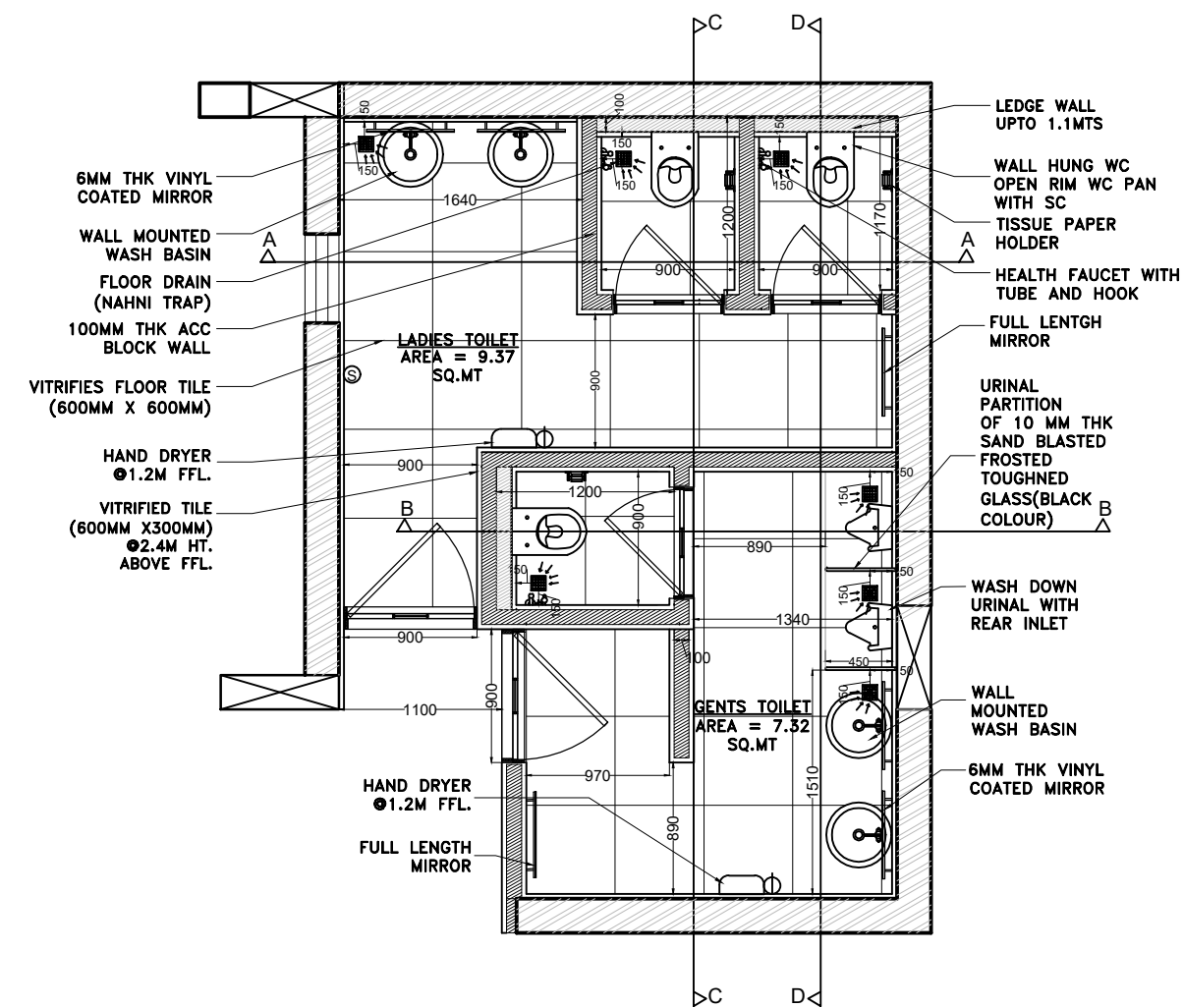
TOILET PLAN SCALE= 1:50
