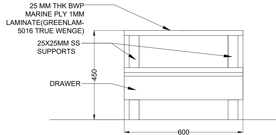
FRONT ELEVATION SCALE= 1:10 (D)
