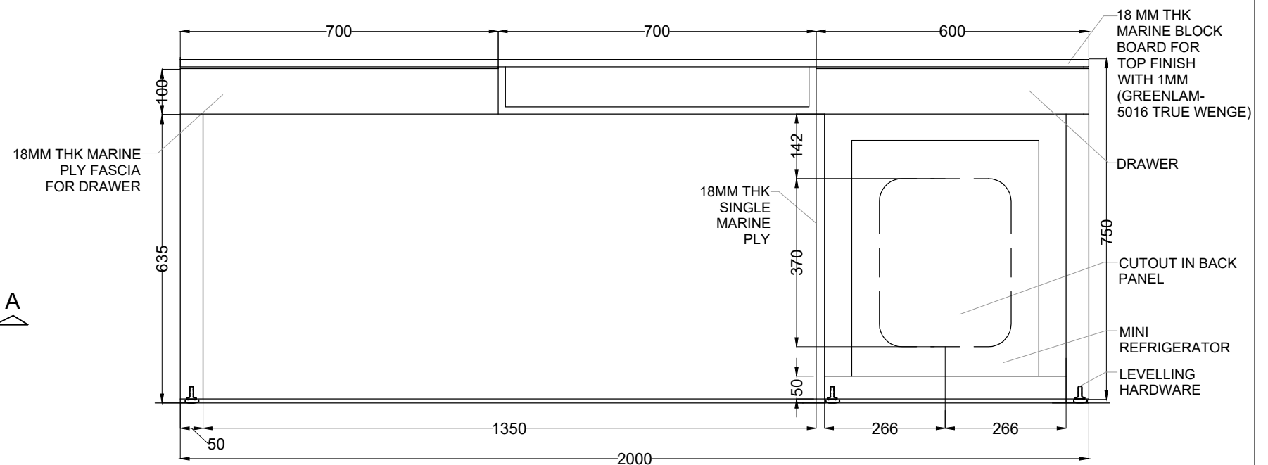
FRONT ELEVATION SCALE= 1:75 (D)
