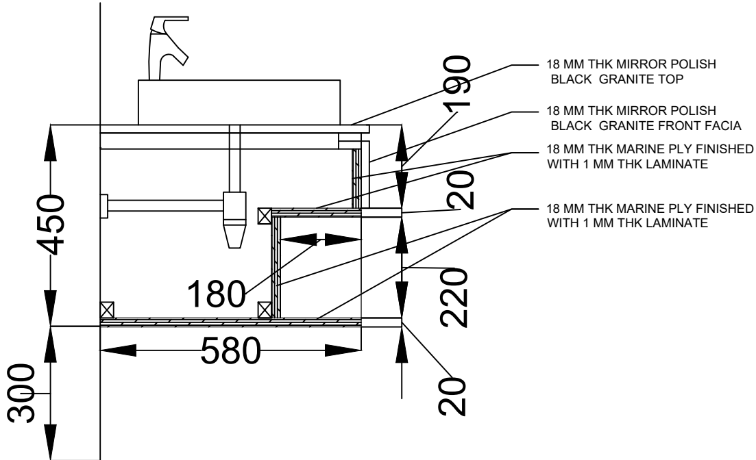
SECTION BB' SCALE=1:15
