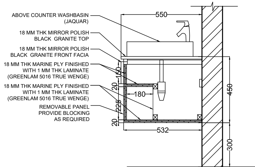
SECTION B-B' (D) SCALE= 1:15
