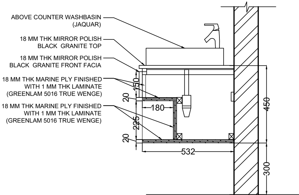
SECTION A-A' (B) SCALE= 1:15
