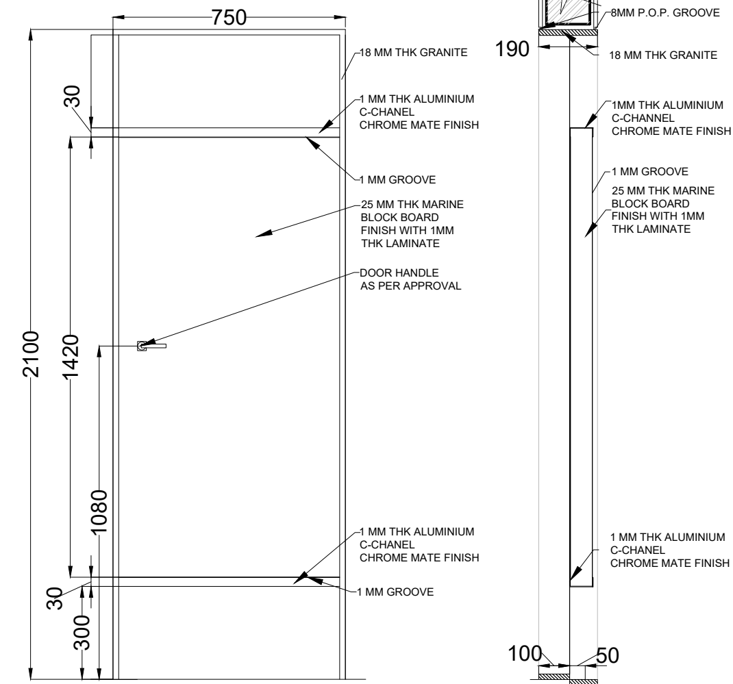
ELEVATION
