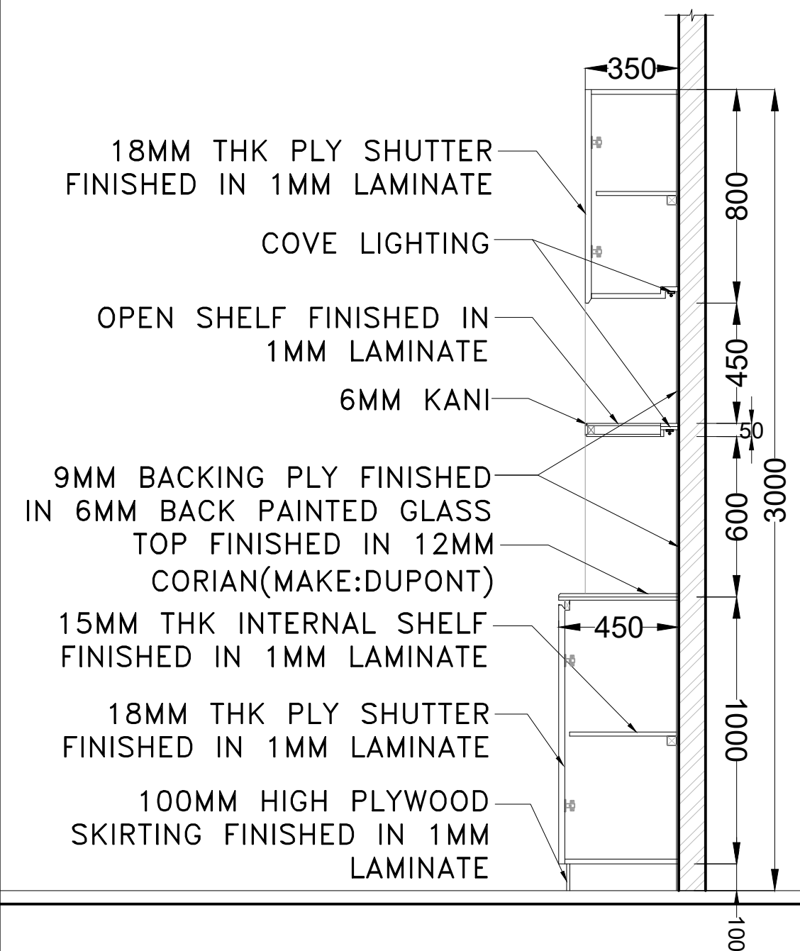
SECTION AA' SCALE= 1:20 (D)
