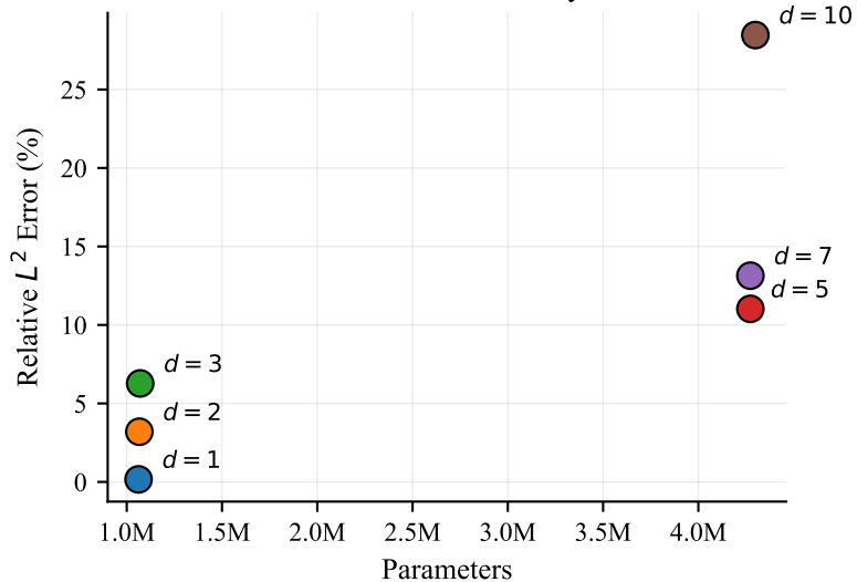
Parameter Efficiency
