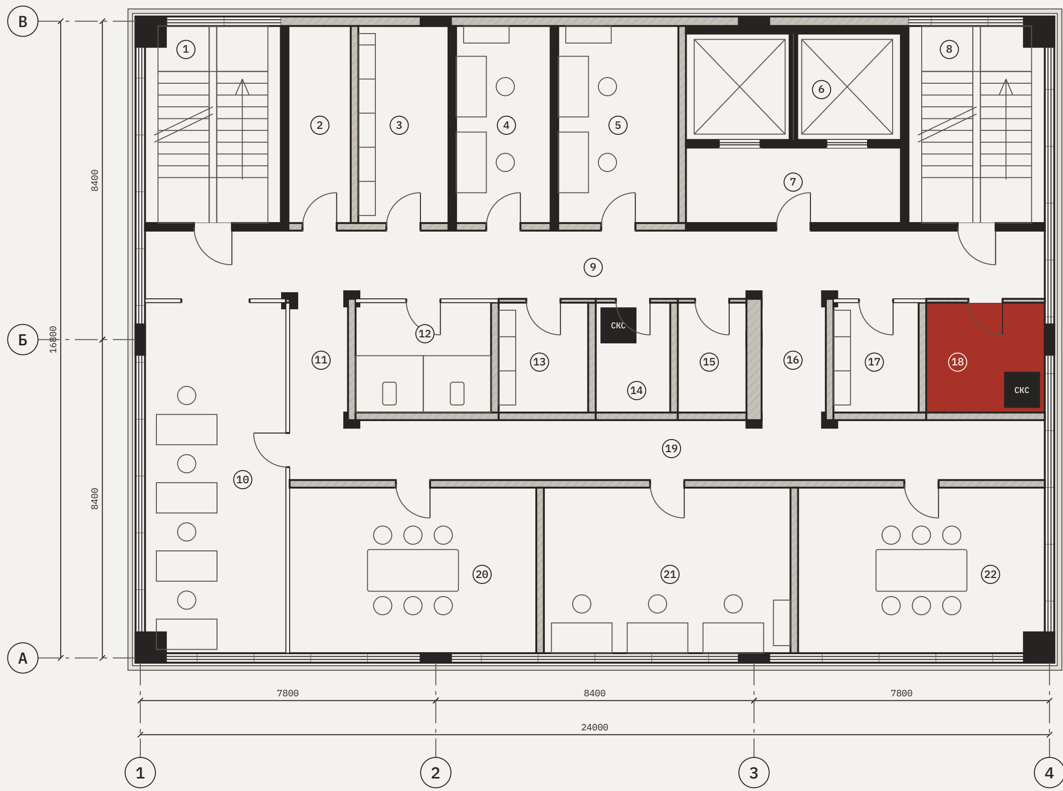
ПЛАН ЭТАЖА НА ОТМ. +0,000 М 1:100
