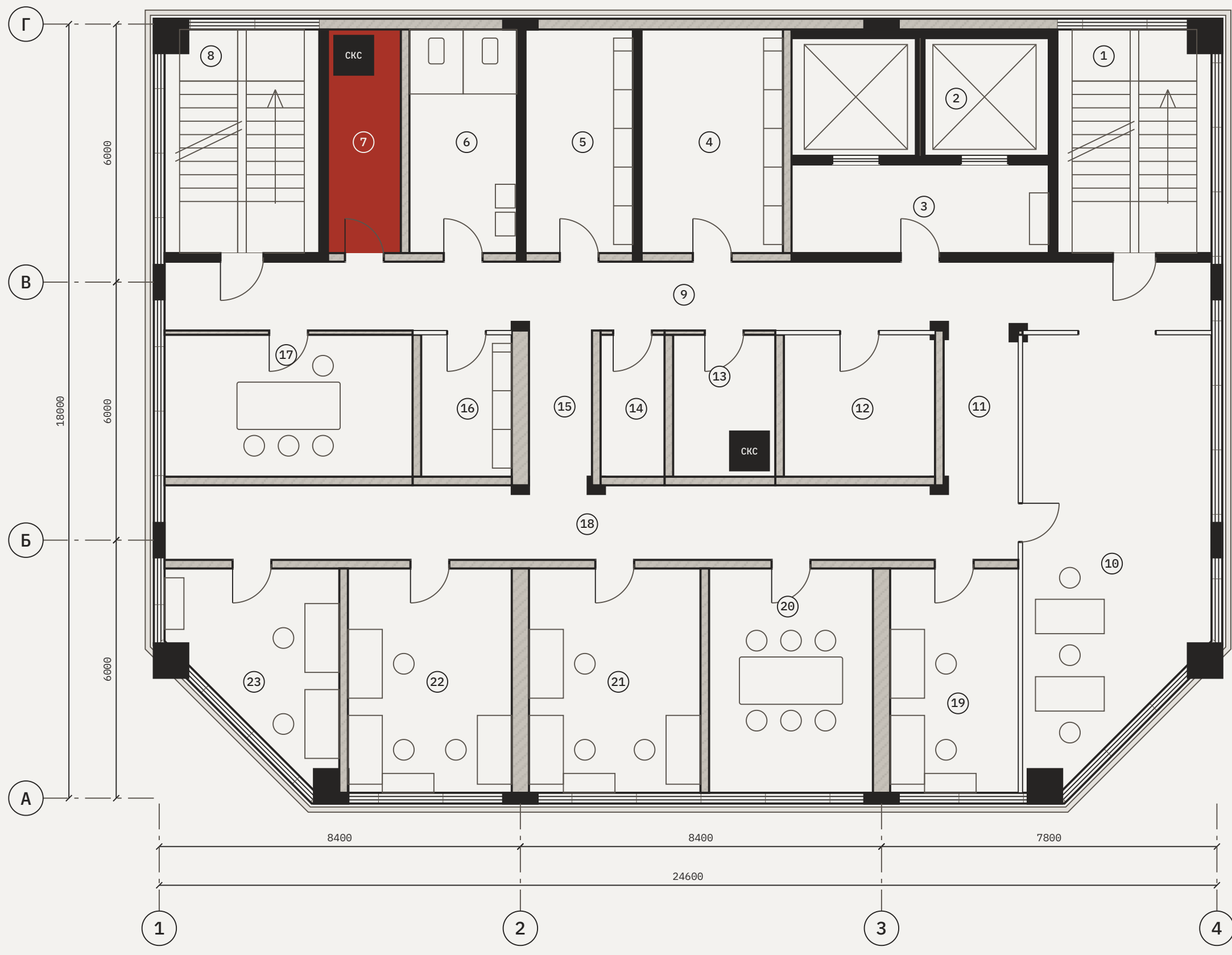
ПЛАН ЭТАЖА НА ОТМ. +0,000
