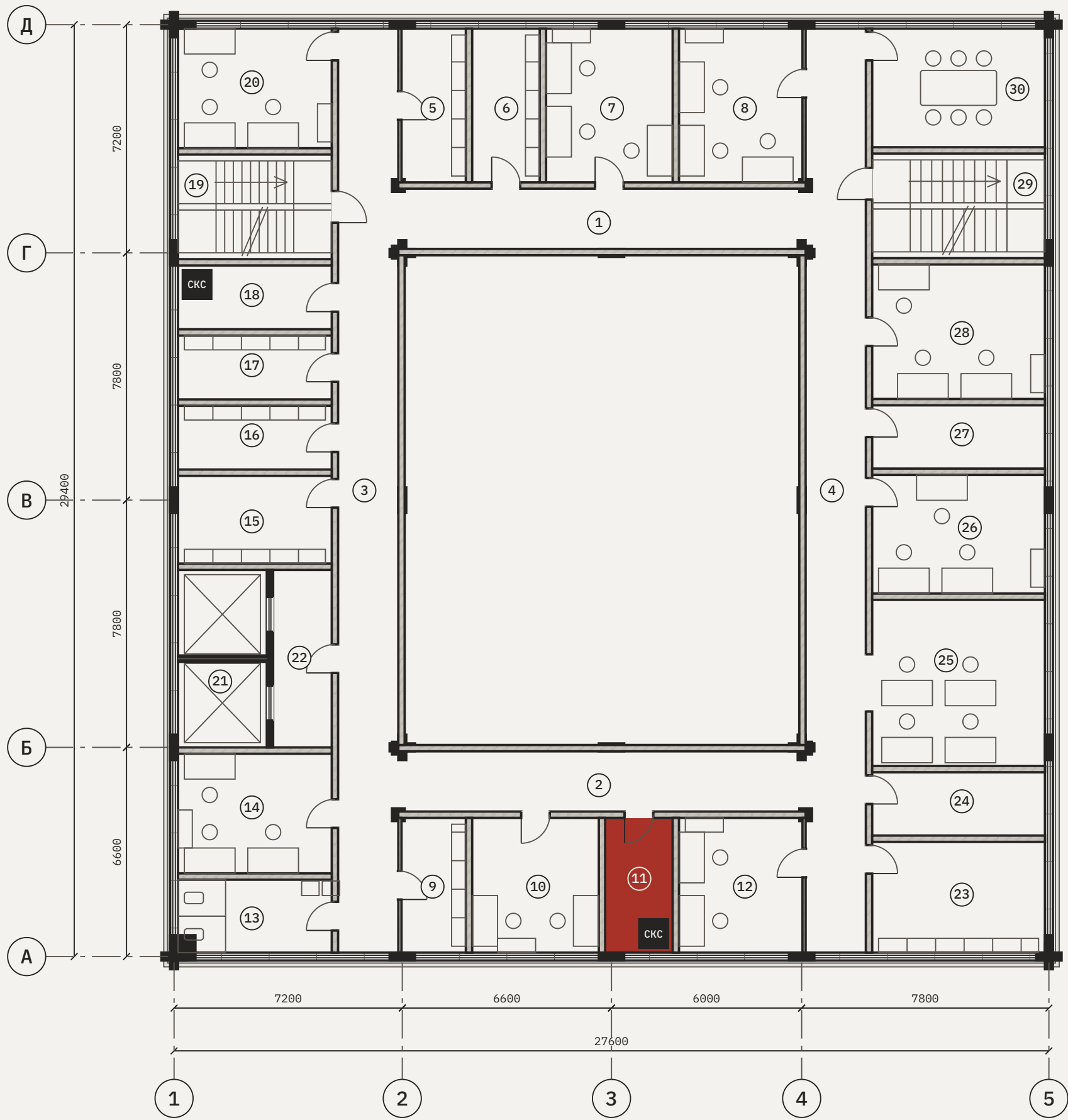
ПЛАН ЭТАЖА НА ОТМ. +0,000 М 1:150
