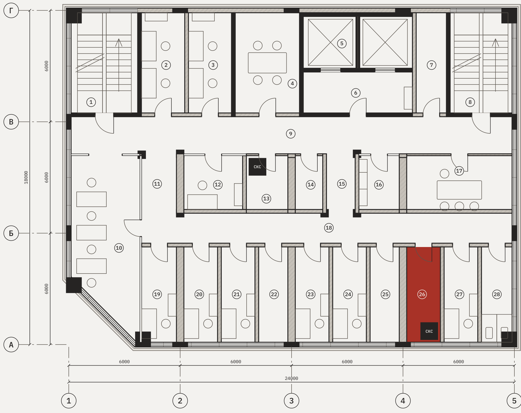
ПЛАН ЭТАЖА НА ОТМ. +0,000 М 1:100
