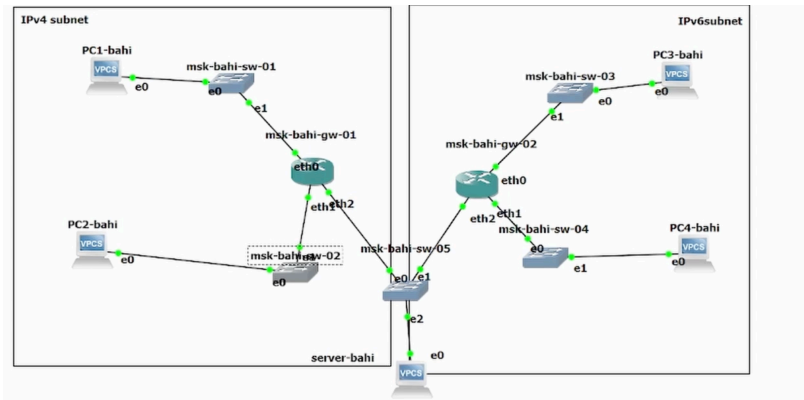
Рисунок 1: Топология сети IPv4 и IPv6
