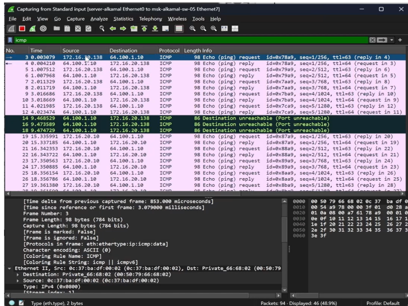
Рисунок 2.17: Детализация ICMP-кадров и информация канального и сетевого уровней
