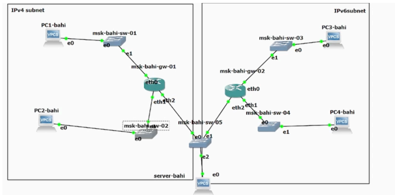
Рисунок 2.1: Топология сети IPv4 и IPv6 в GNS3 с маршрутизаторами FRR и VyOS
