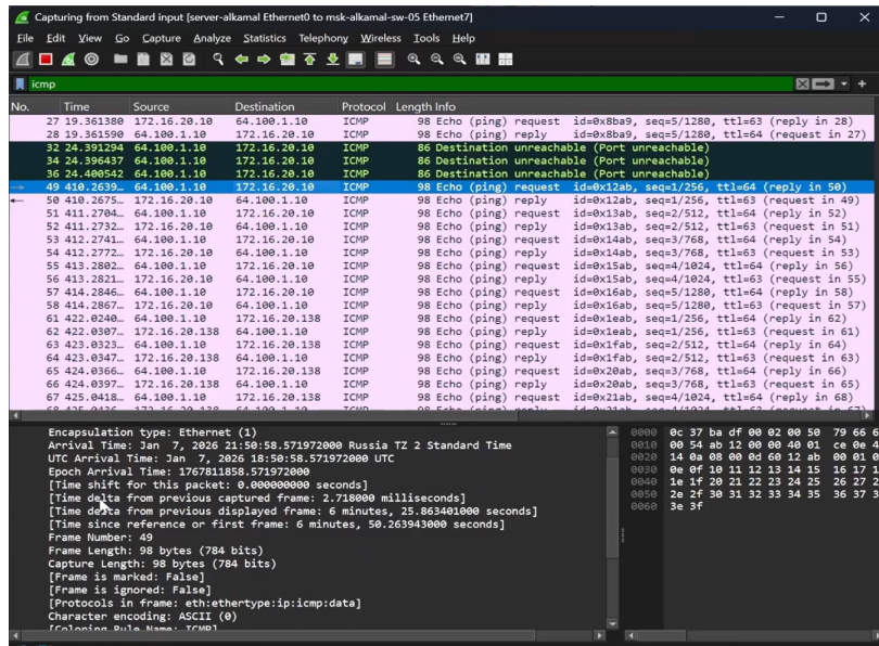
Рисунок 2.16: ICMP-трафик IPv4 между сервером двойного стека и узлами подсети
