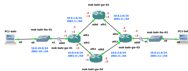
Рисунок 2.1: Топология моделируемой сети в GNS3 с четырьмя маршрутизаторами и окончными узлами
