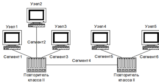
Рис. 2.4. Топология сети
