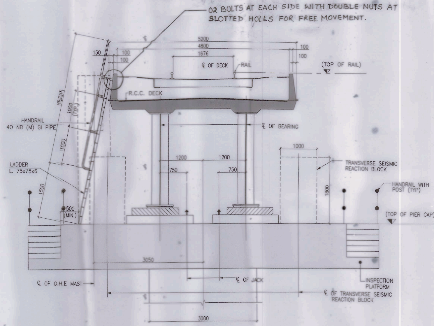
SECTION A-A (SCALE 1:40)
