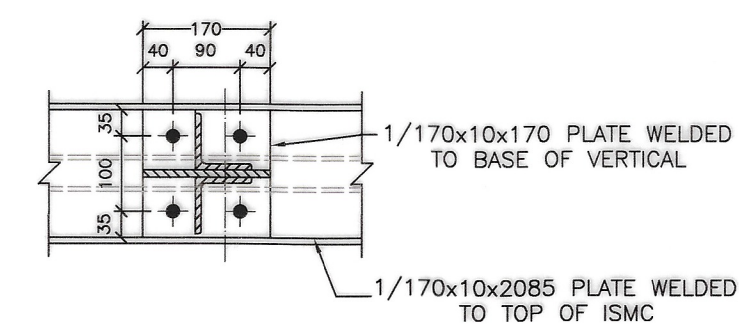
PLAN D-D (SCALE-1:10)
