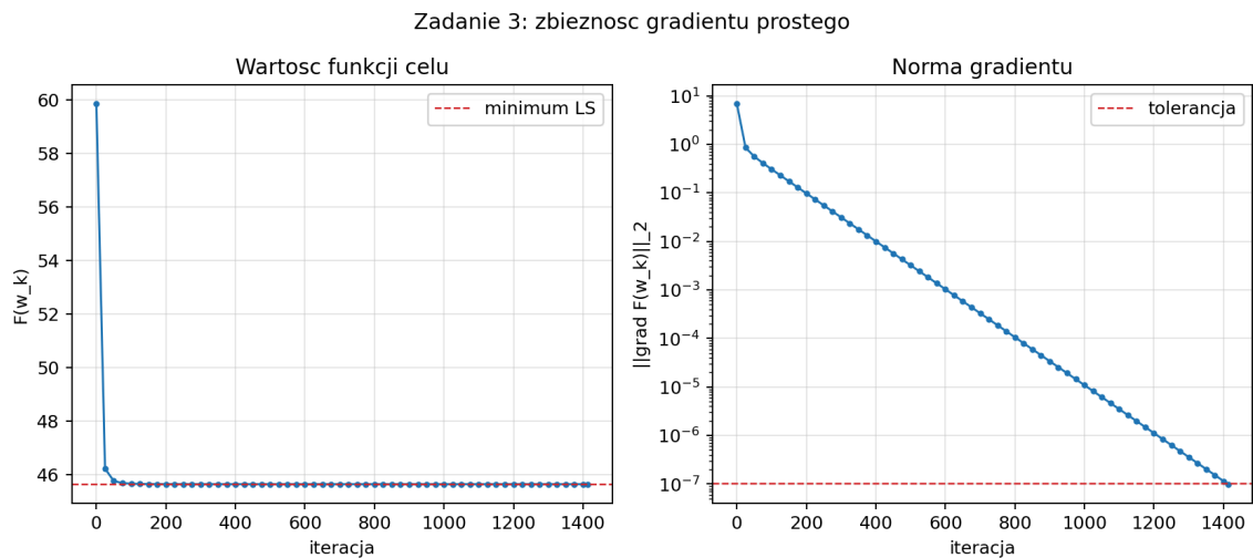
Figure 5: Zbieżność gradientu prostego: wartość funkcji celu oraz norma gradientu z zaznaczoną tolerancją stopu.
