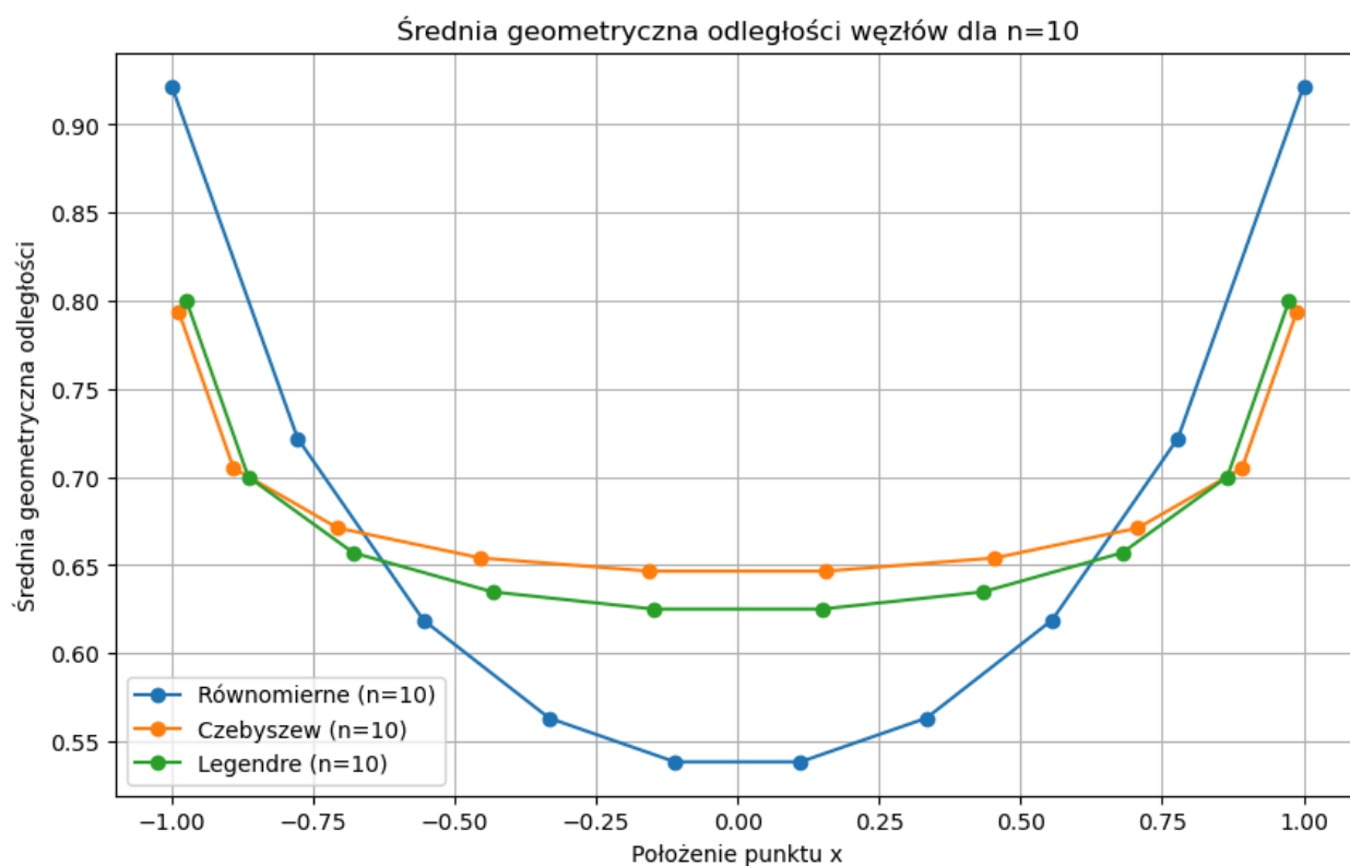
Rysunek 1: Średnia geometryczna odległości węzłów interpolacji dla punktów równomiernych, Czebyszewa i Legendre'a przy n = 10 .
