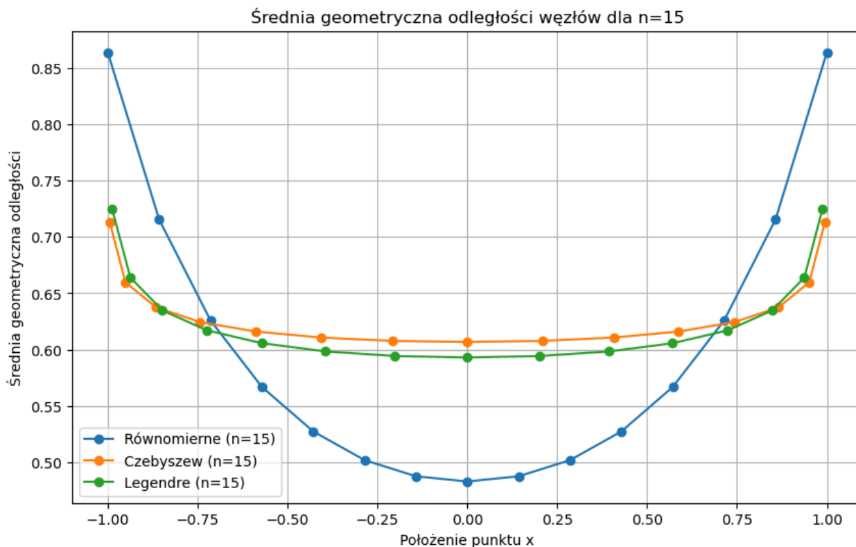
Rysunek 1: Średnia geometryczna odległości węzłów interpolacji dla punktów równomiernych, Czebyszewa i Legendre'a przy n = 15 .
