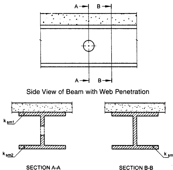
FIG. 26 WEB PENETRATION
