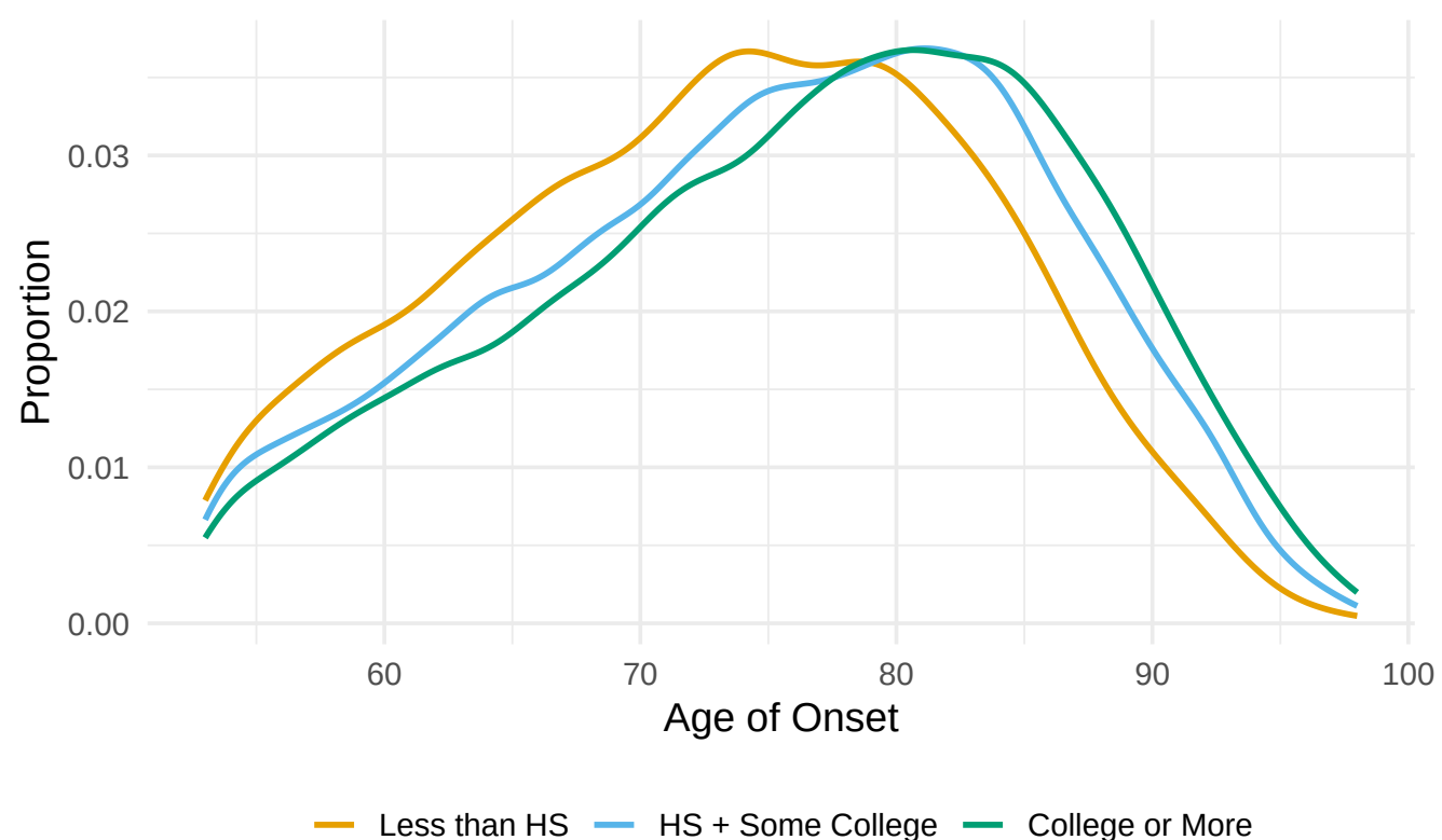
(D) Educational Attainment
