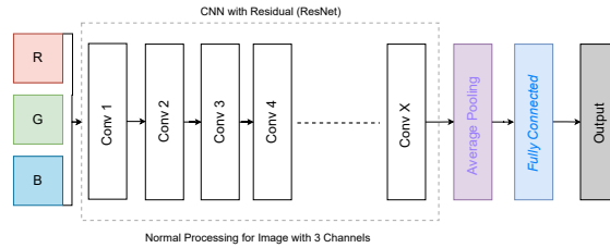
Gambar 3.6 Arsitektur ResNet dua dimensi untuk klasifikasi gambar input RGB
