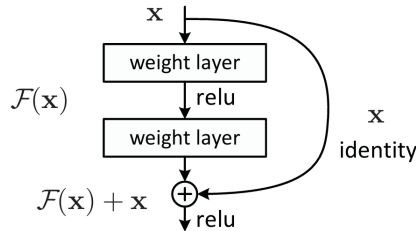
Gambar 2.7 Struktur blok residual pada Residual Network (ResNet)
