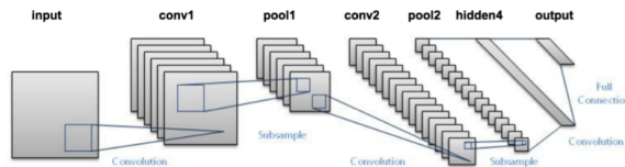
Gambar 2.5 Arsitektur dasar CNN dua dimensi Sumber: diadaptasi dari LeCun et al. [34]
