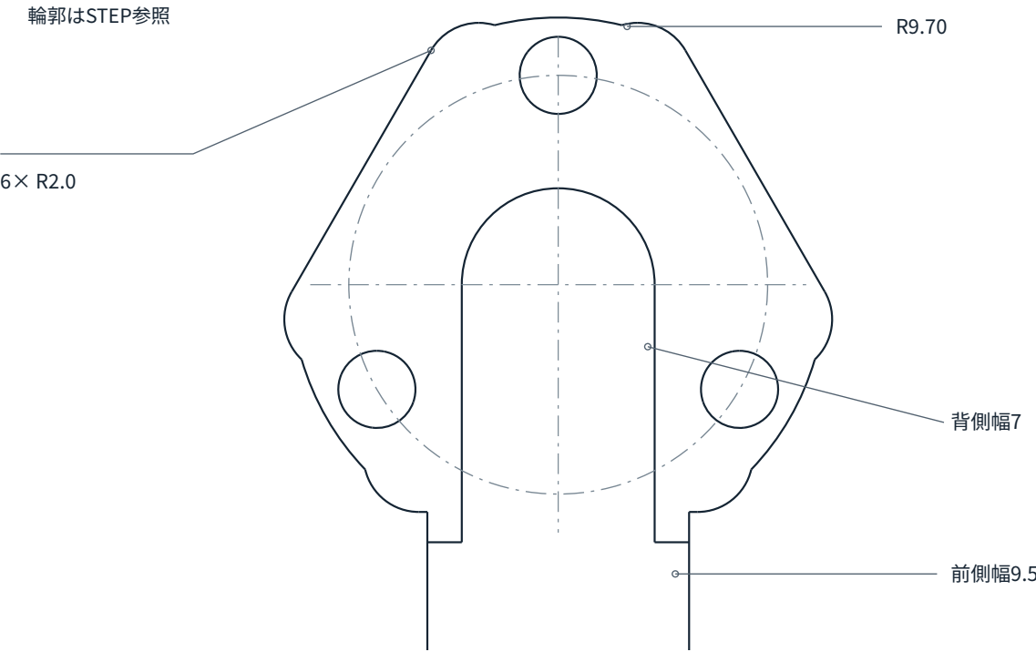
受け部詳細 4:1
