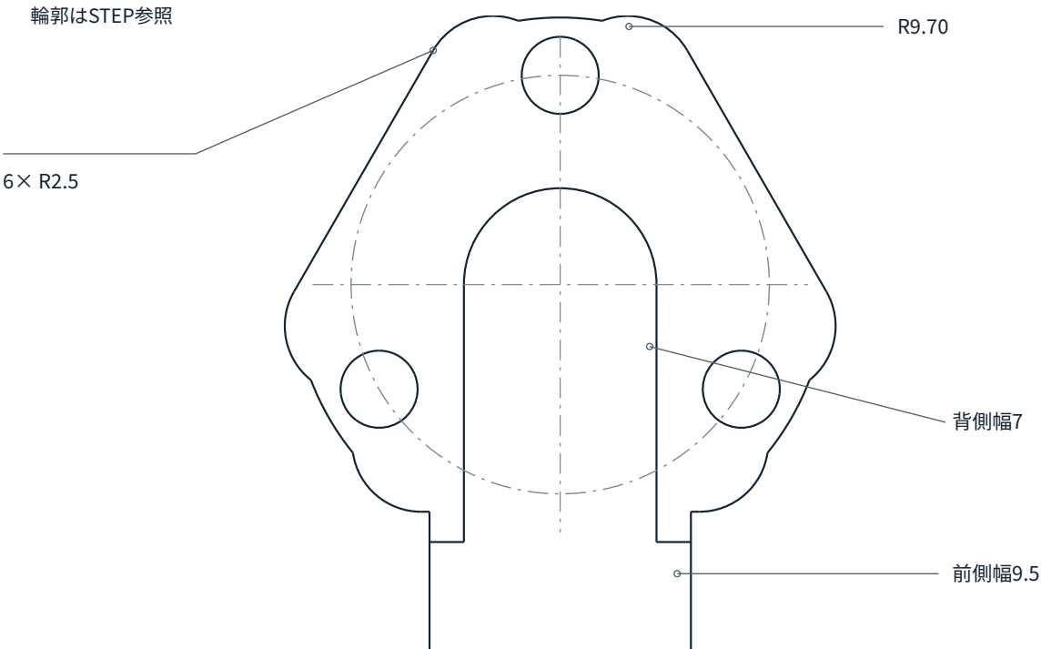
受け部詳細 4:1
