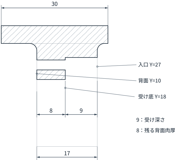
軸中心 X=45 の断面 2:1 薄灰色は外形投影。下側は配線開口。
