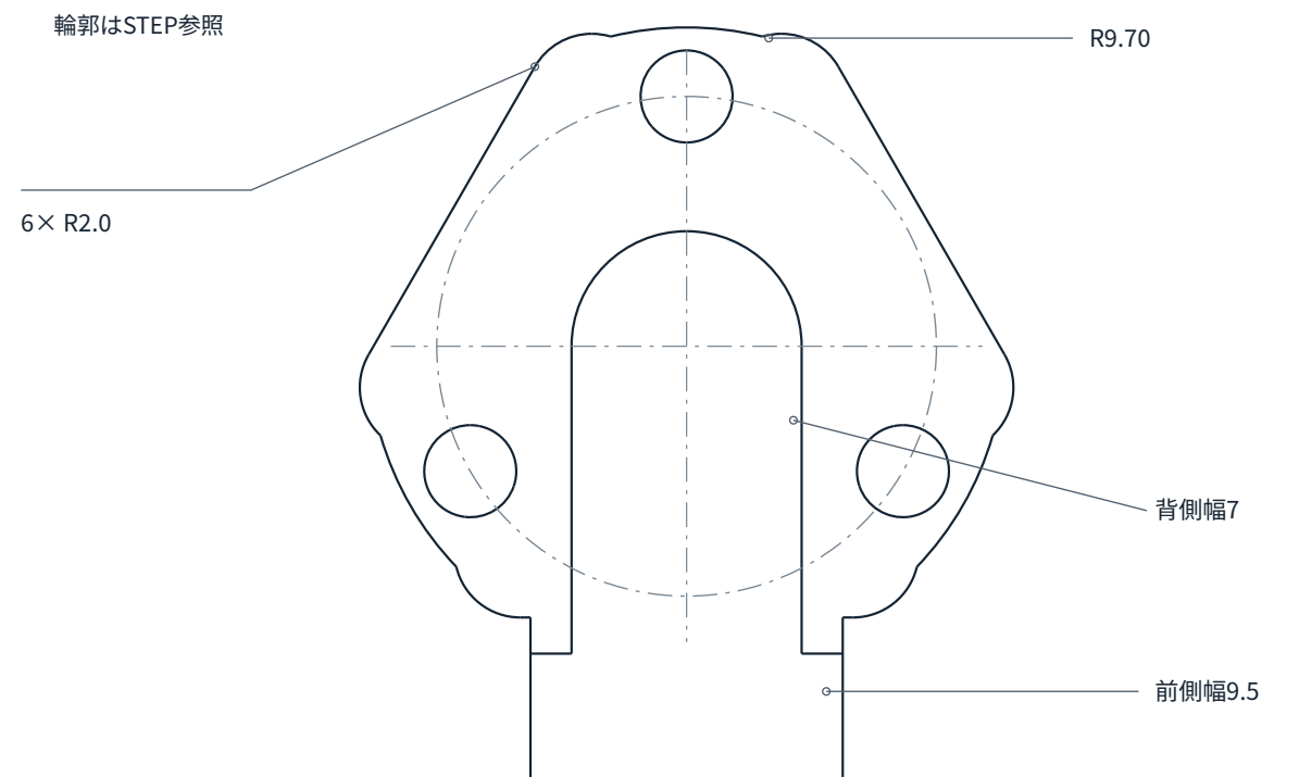
受け部詳細 4:1
