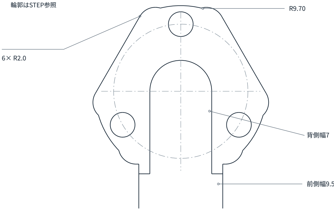
受け部詳細 4:1
