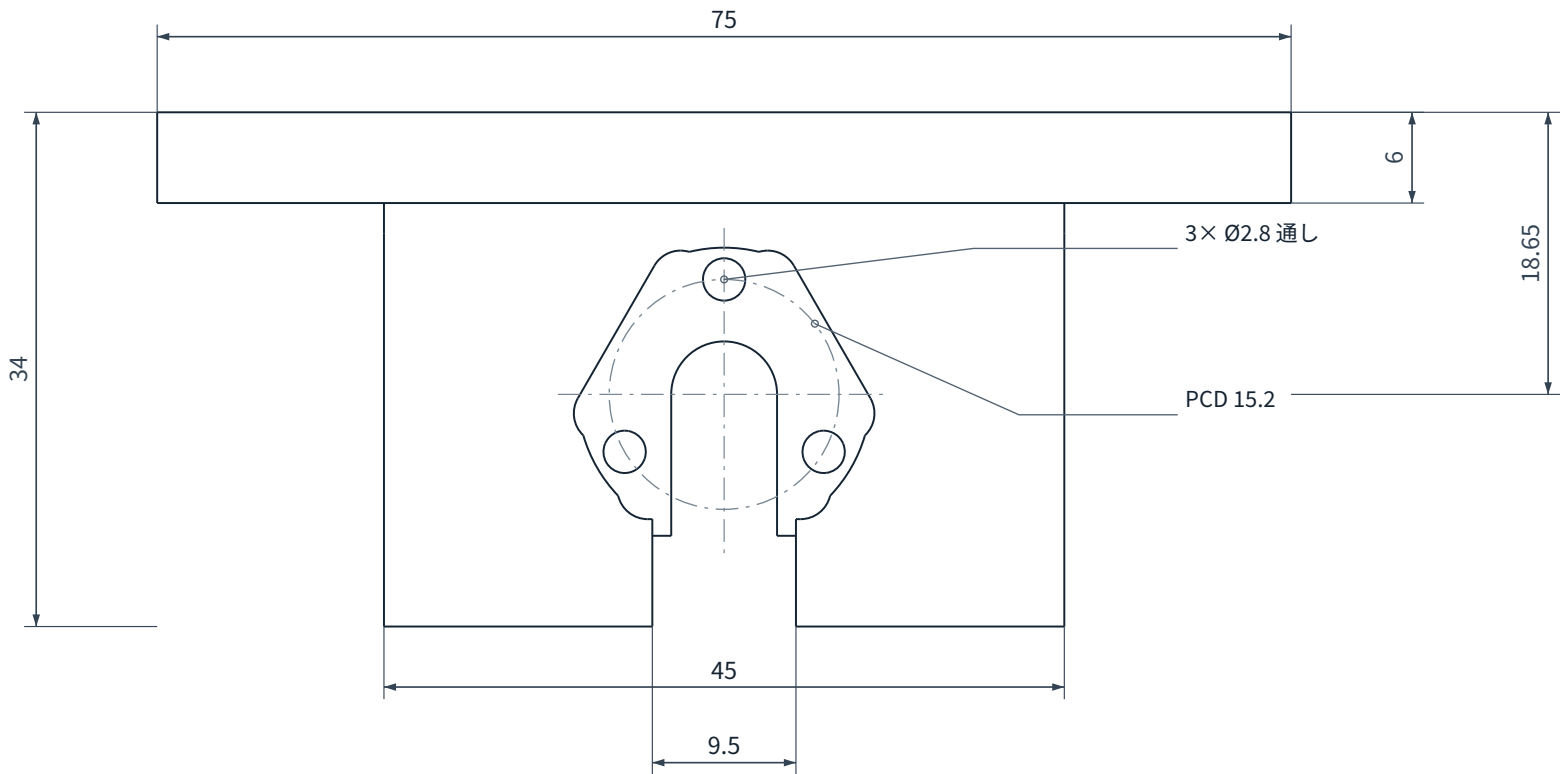
モータ側正面（+Y側から） 2:1
