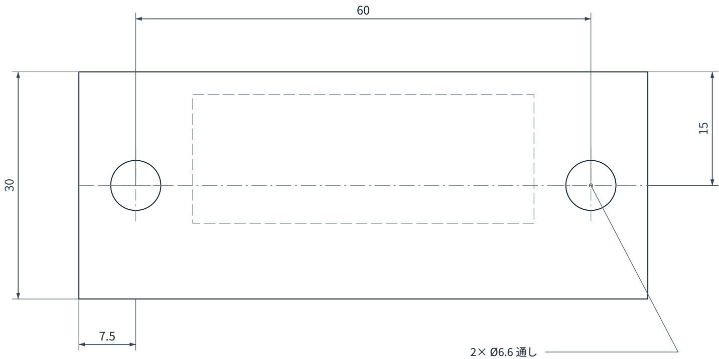
3030接触面（+Z側から） 2:1
