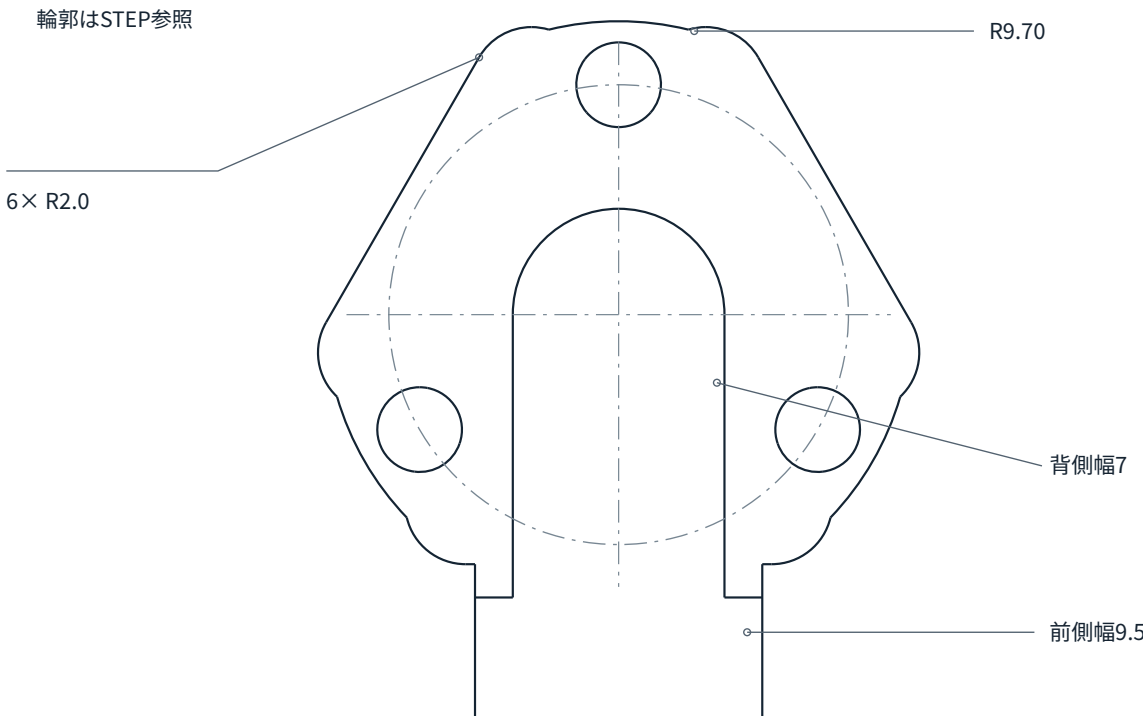
受け部詳細 4:1
