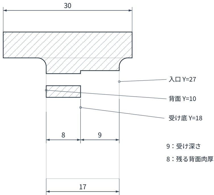
軸中心 X=37.5 の断面 2:1
