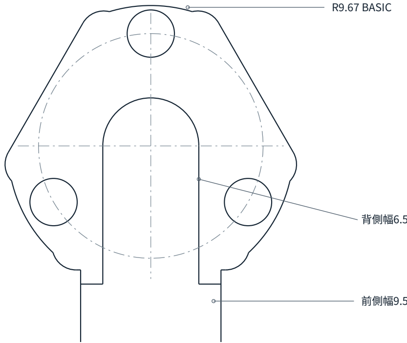
受け部詳細 4:1
