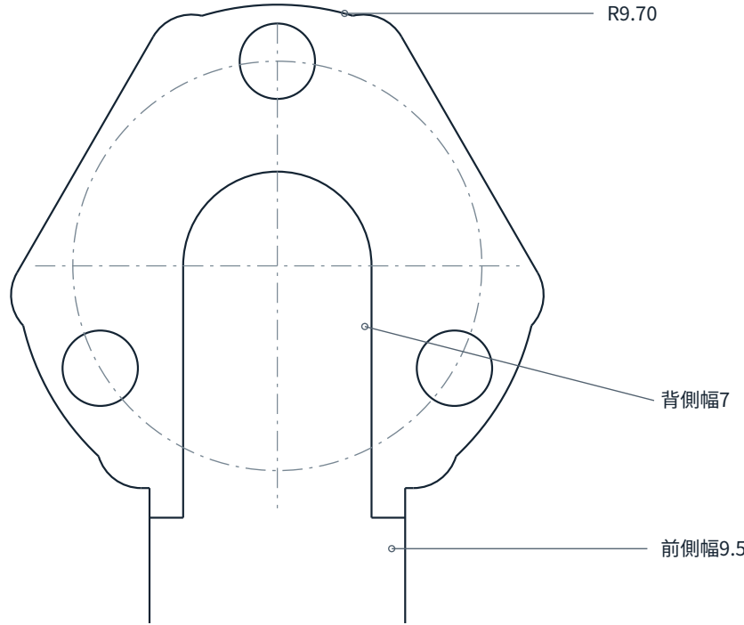
受け部詳細 4:1
