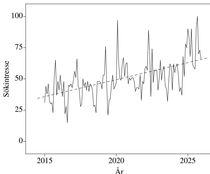
Figur 3. Googles sökintrasse för sökfrasen Antonio Gramsci 2015–2025 i USA (relativt index, 100 = högsta värdet i perioden). 11
