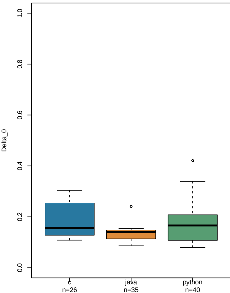
Token multiset Dice
