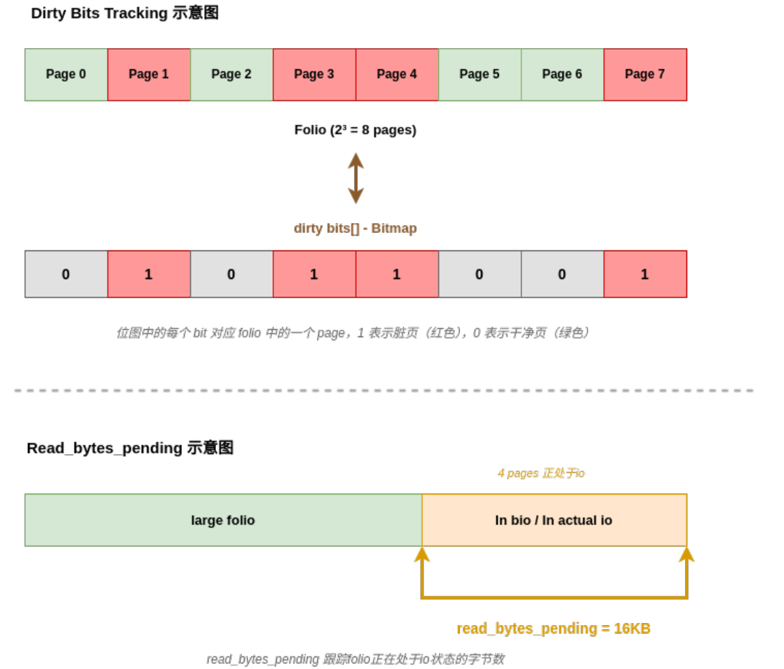
图 2-7 iomap 动态大页状态对象中的逐块位图与 pending 计数
