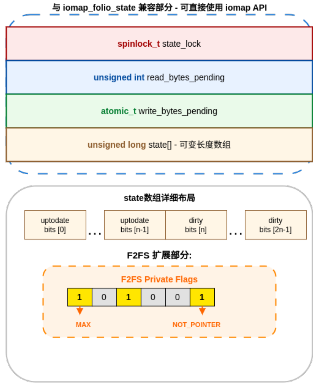
图 3-2 F2FS 扩展型动态大页状态对象布局
