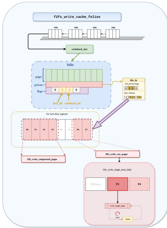
图 4-4 动态大页脏区间写回路径
