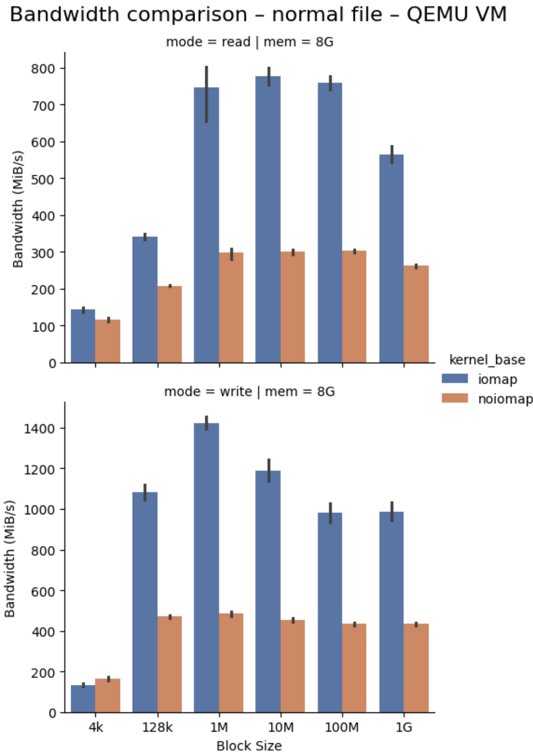
图 5-1 QEMU 平台普通文件顺序 I/O 带宽对比
