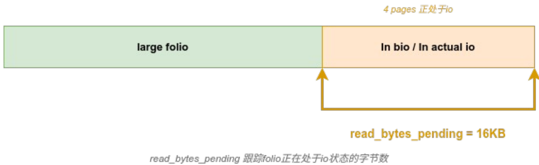
图 4-6 未完成读字节计数的偏置等待机制
