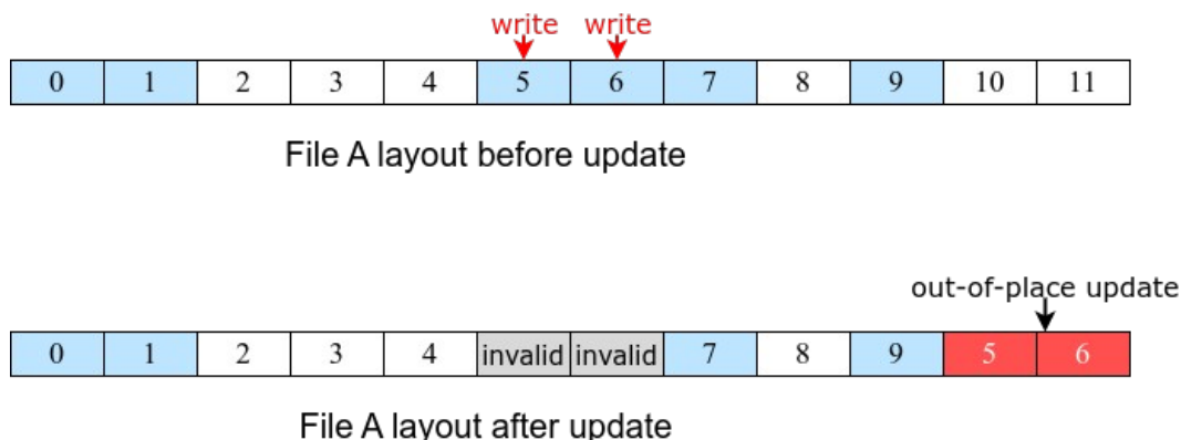
图 2-4 F2FS 异地更新过程示意
