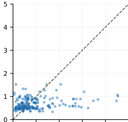
Affine BVSE MAE = 0.296 eV
