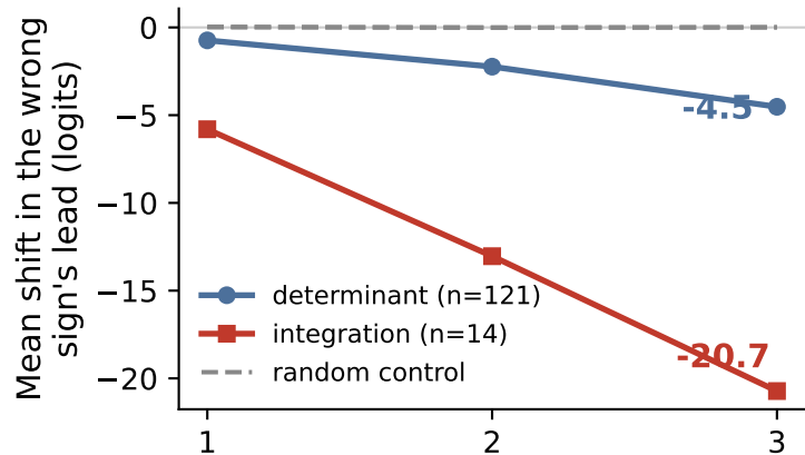
Llama-3.3-70B — steer L77+L79
