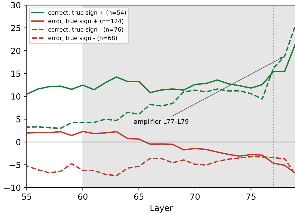
Llama-3.3-70B
