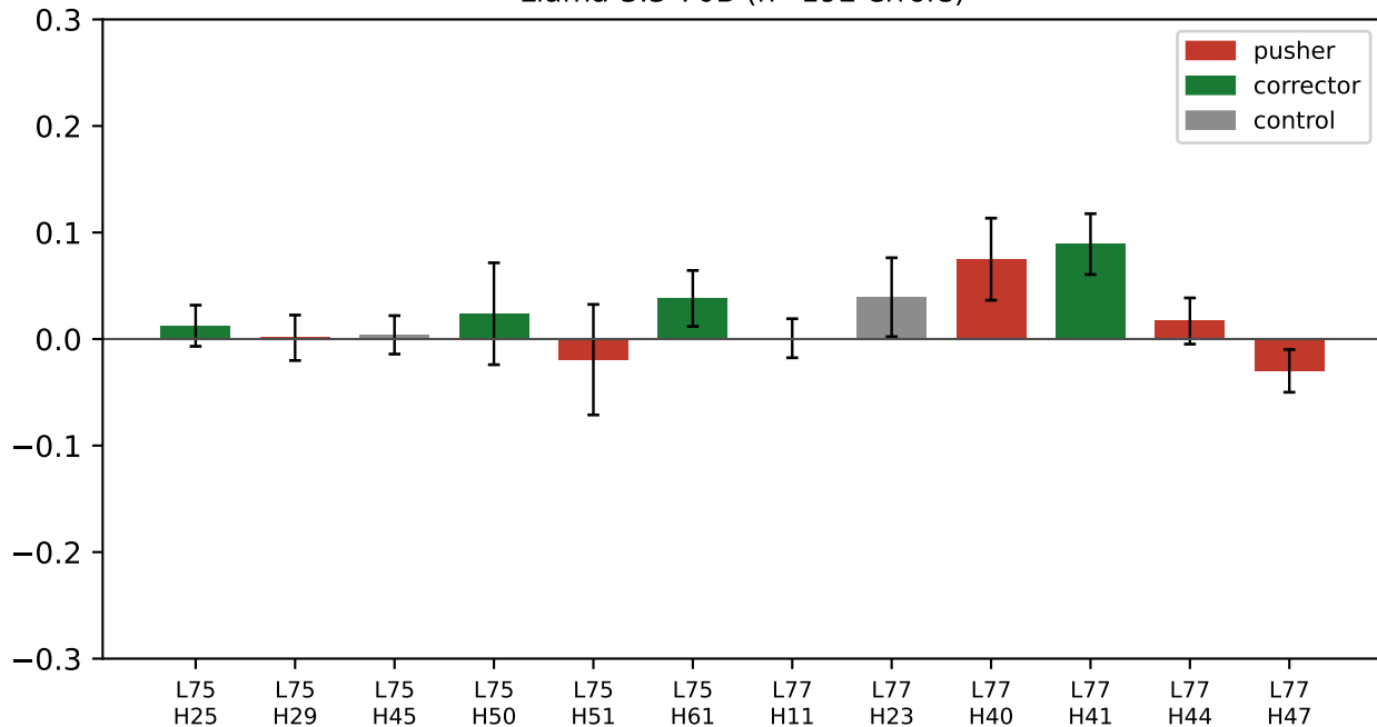
Llama-3.3-70B (n=192 errors)
