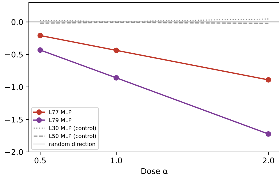
Llama-3.3-70B (n=189 errors)
