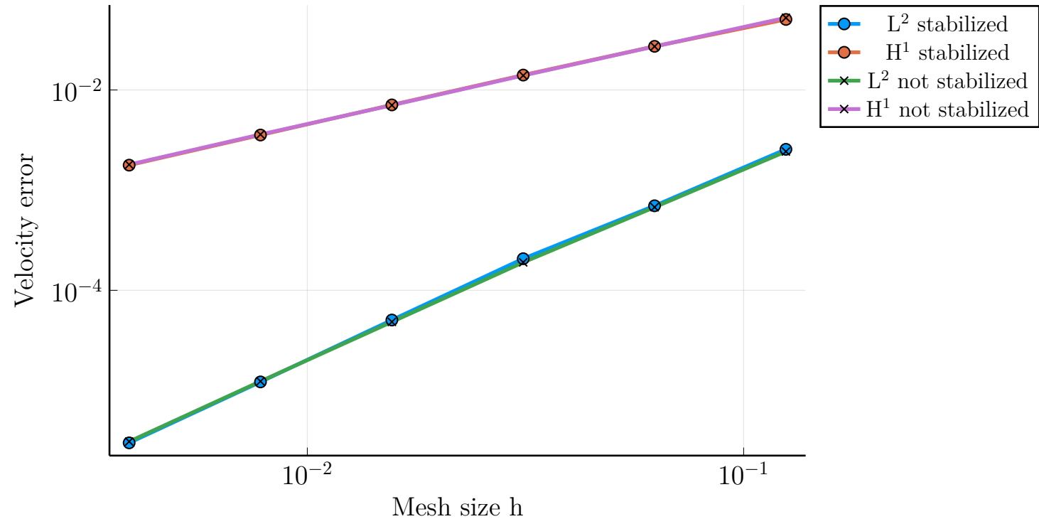
Convergence Poisson
