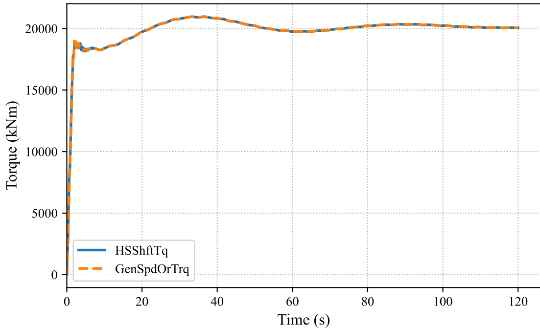
HSShftTq vs GenSpdOrTrq
