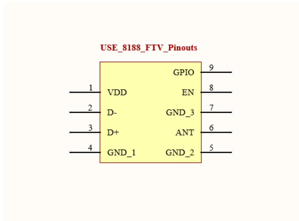
Fig1: Module Pinouts
