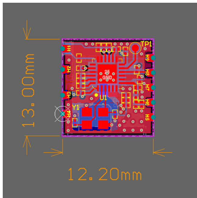
Fig 3 : Module dimension drawing
