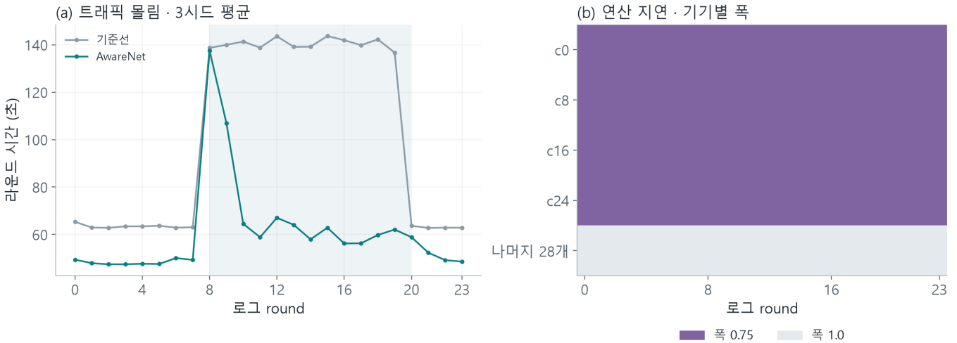
그림 6. 트래픽 몰림의 시간 응답과 연산 지연 기기의 폭 선택
