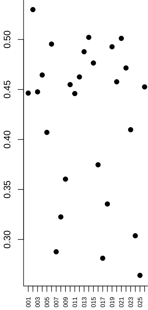
correlacao ponto-biserial
