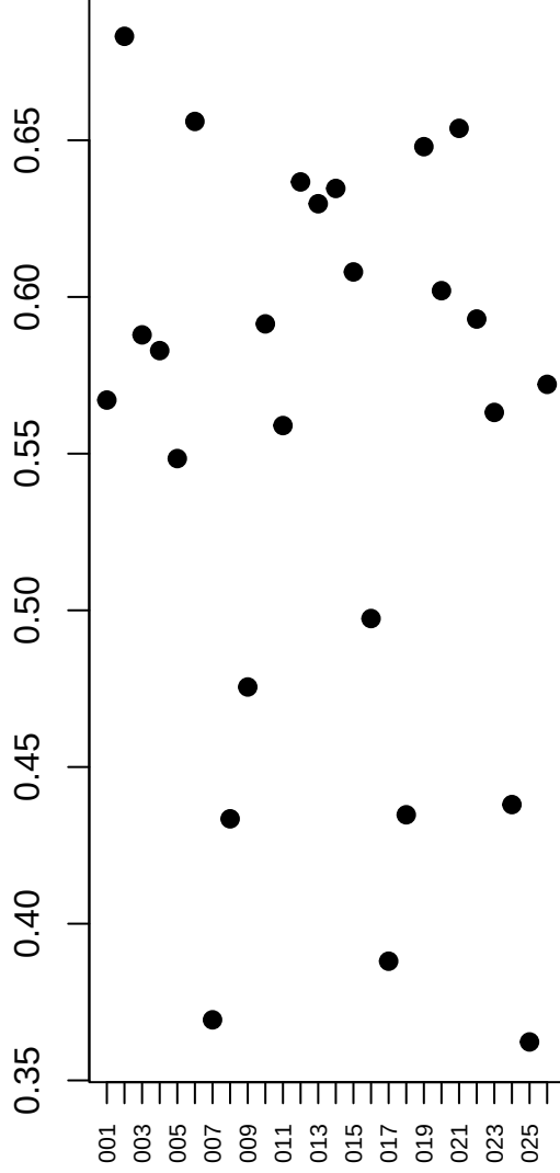
correlacao biserial
