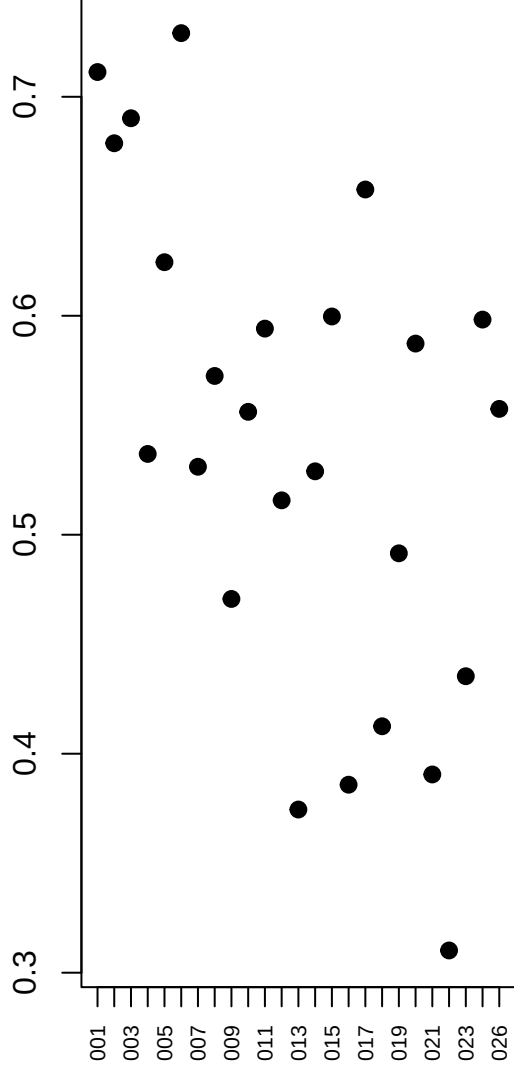
correlacao bisserial
