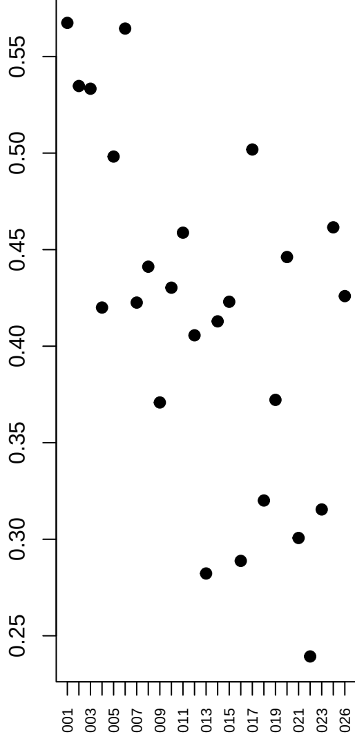
correlacao ponto-bisserial
